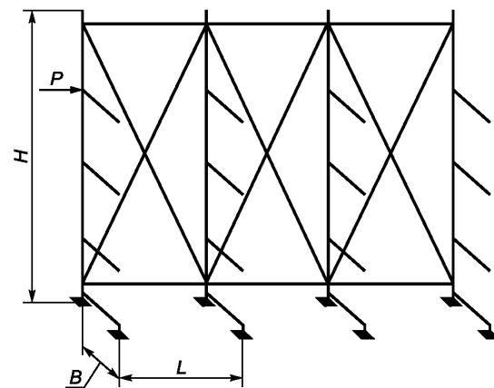
Консольный стеллаж
