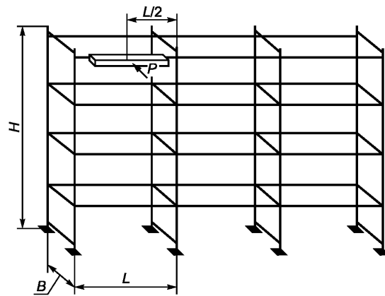
Фронтальный стеллаж
