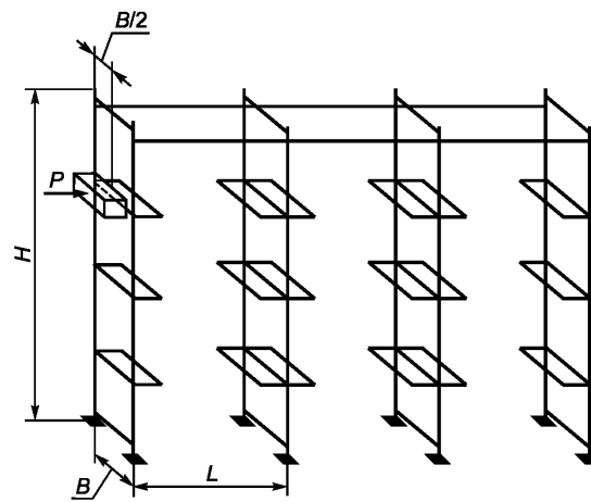
Глубинный стеллаж
