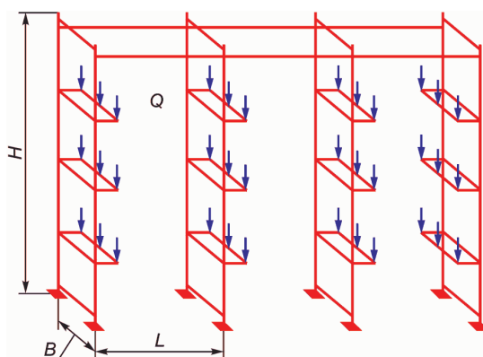
Глубинный стеллаж
