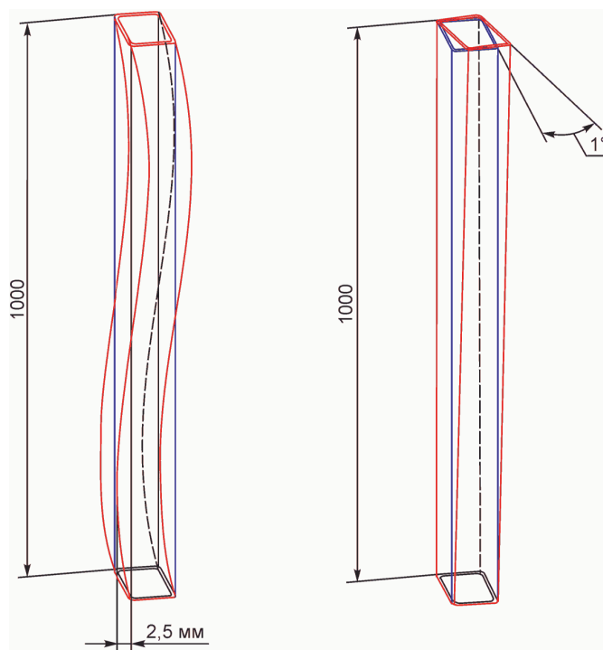
Рисунок 4 - Кривизна и скручивание стоек
