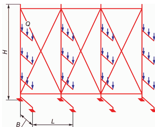
Консольный стеллаж
