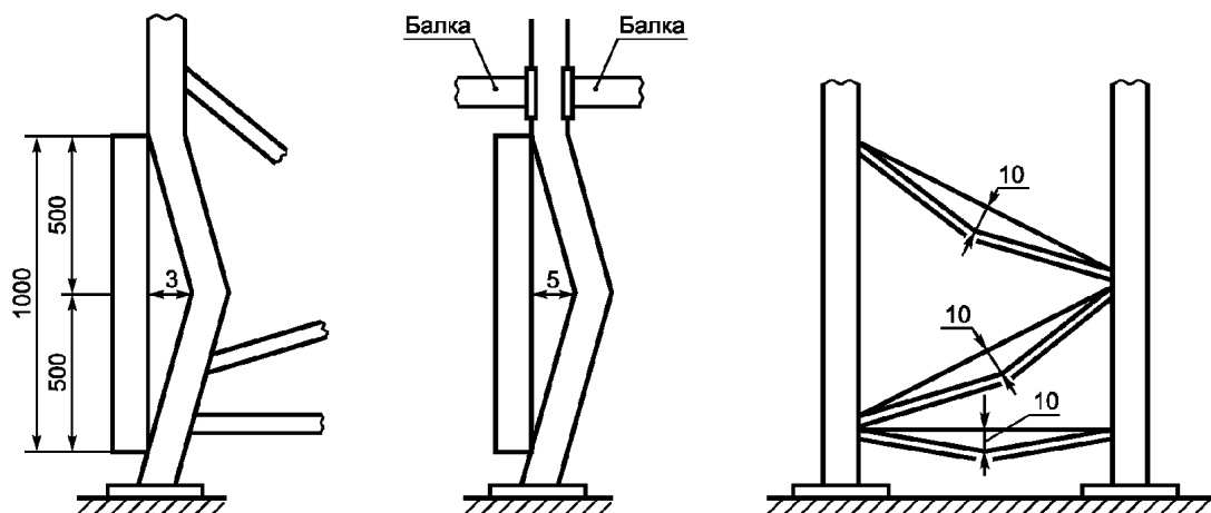
Рисунок Б.1 - Максимальные допустимые значения деформации
