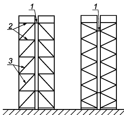
1 - межрамная связь; 2, 3 - элементы раскосной системы
