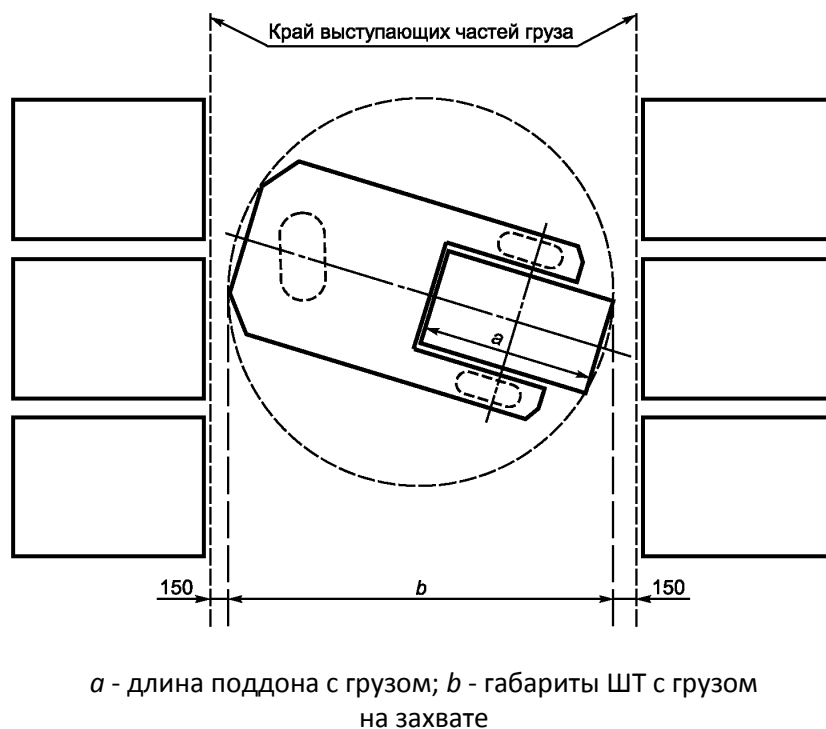
Рисунок 5 - Параметры зазора между ШТ и грузами
